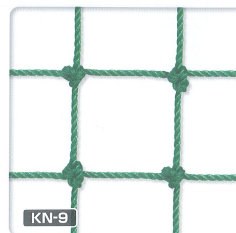
ポリエチレン 440T/30本 目合 25mm グリーン
