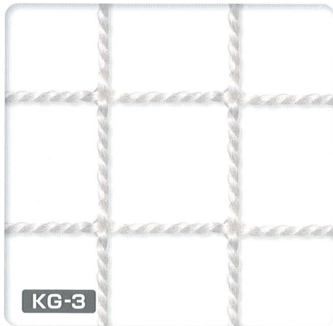
ポリエチレン 440T/36本 目合 25mm 白
